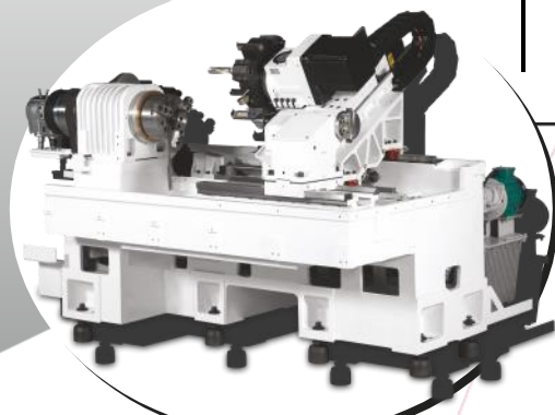
DX 200 Struktur Struktur mit starrem Bett und einem einteiligen, um 30° geneigten Schlitten, der hohe Schnittkräfte und eine schnellere Produktion zulässt.
