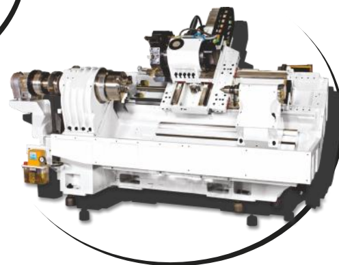
DX 350 Struktur Einteilige Struktur mit starrem 45°-Bett, das selbst in harten Materialien große Schnitte zulässt.
