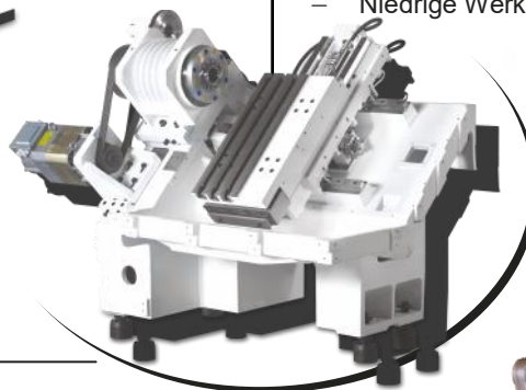
DX 350 Struktur Einteilige Struktur mit starrem 45°-Bett, das selbst in harten Materialien große Schnitte zulässt.
